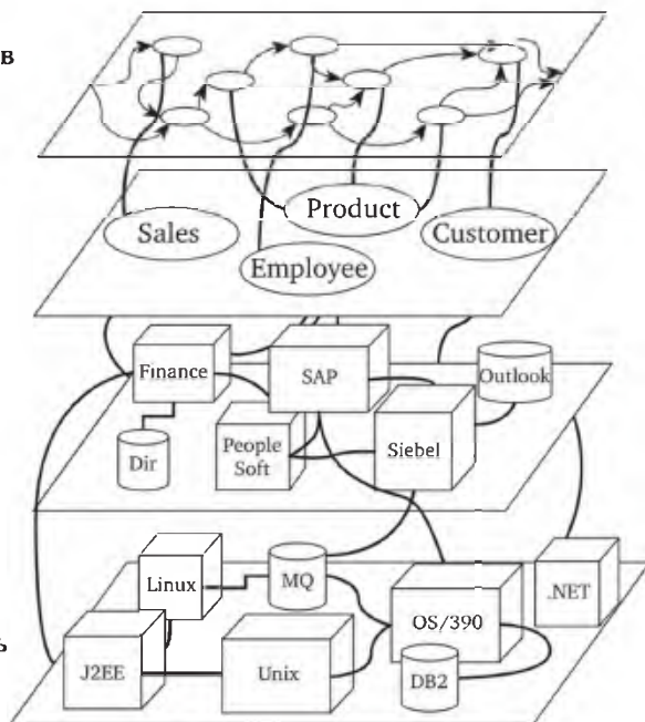
Рис. 3.36. Иллюстрация роли сервисов как уровня взаимодействия между ИТ и бизнесом в концепции SOA
