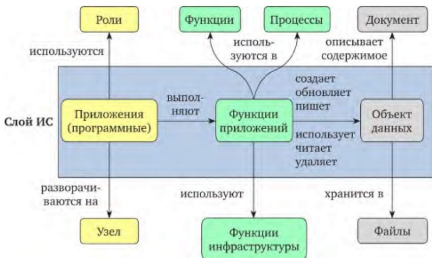
Рис. 3.30. Связи между объектами (мета модель) слоя ИС
